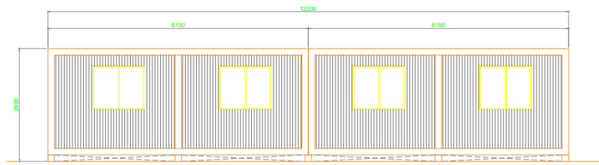
2 FRONT ELEVATION SCALE: 1:20m
